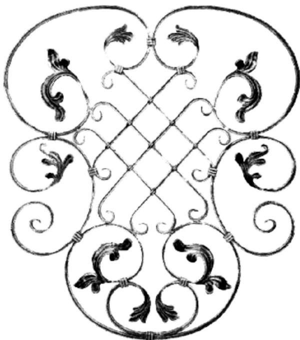
13.029.16 13.029.14 Baza: 16x6 mm Baza: 14x6 mm H: 700 mm H: 700 mm L: 800 mm L: 800 mm
