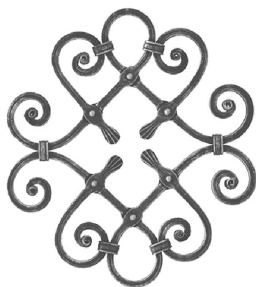
13.019 Baza: 12x12 mm H: 460 mm L: 410 mm
