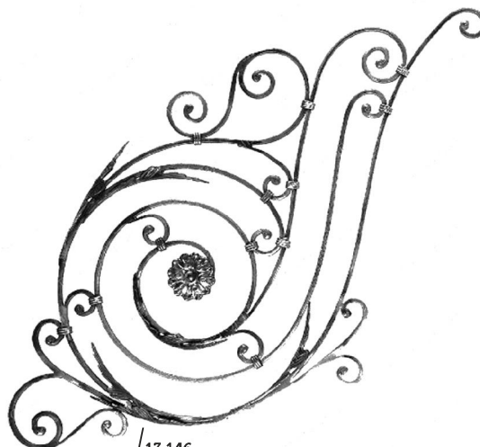
13.146 Baza: 16x8 mm H: 840 mm L: 770 mm
