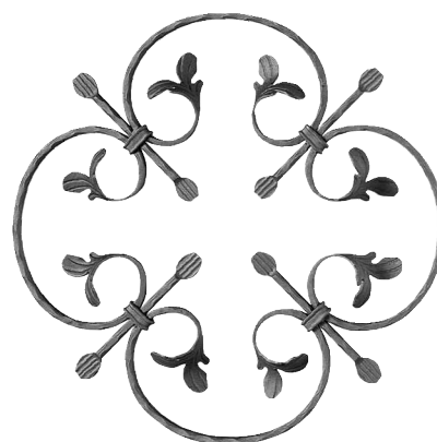
13.071 Baza: 12x6 mm H: 410 mm L: 410 mm Amprentat
