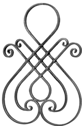
13.024.06 Baza: 16x6 mm H: 575 mm L: 410 mm
