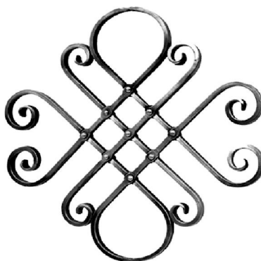
13.021 Baza: 16x8 mm H: 400 mm L: 410 mm
