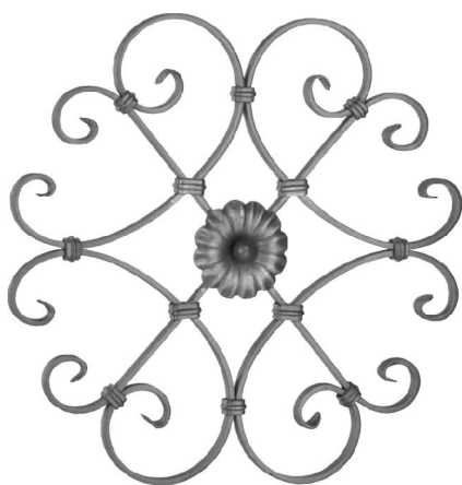
13.016.08 Baza: 16x8 mm H: 480 mm L: 410 mm
